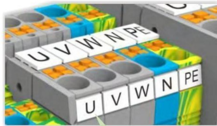
侧面标记区 Side marking area
